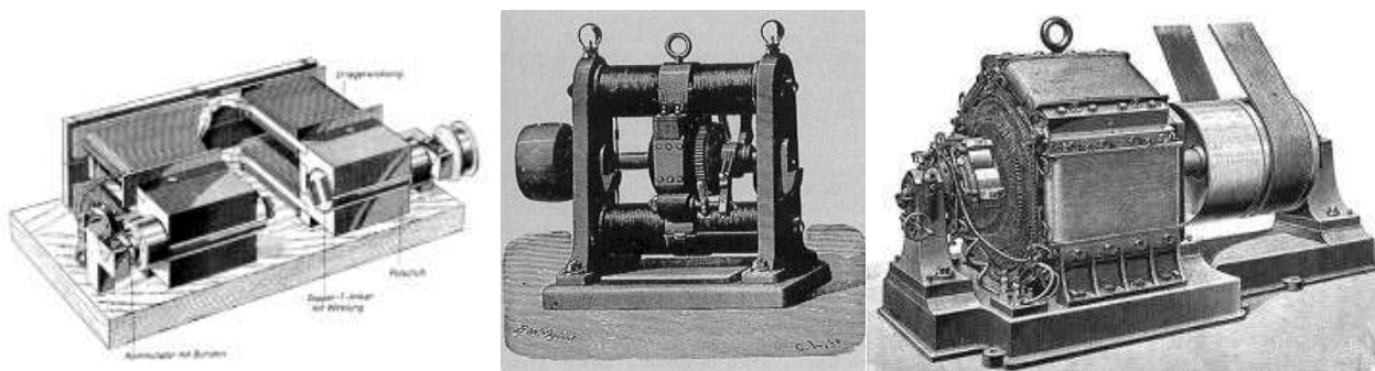
Dínamo de Siemens 5 (esq.) e de Gramme (dir) 6 e dínamo de seis polos 7 patenteado por René Thury em 1883 (abaixo).
