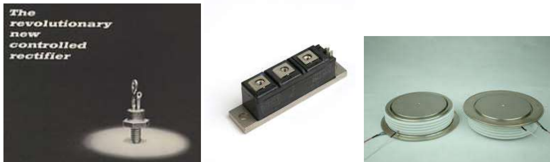
Publicidade do primeiro SCR (Tiristor) pela GE 28 e dispositivos modernos
